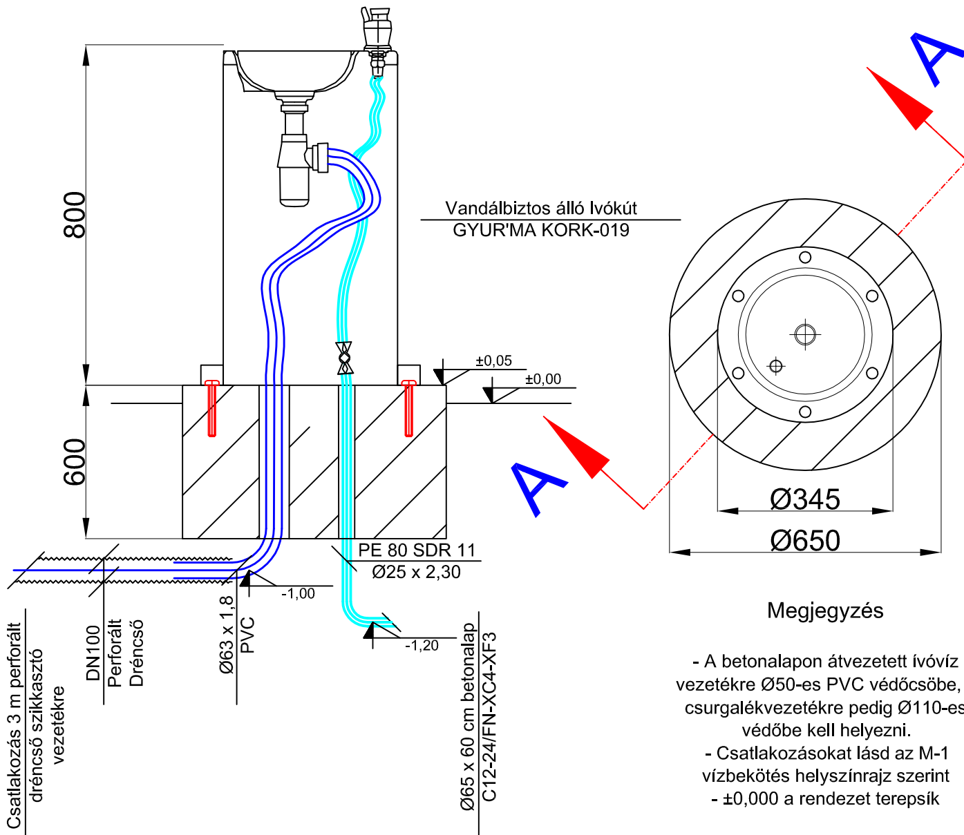
Ivókút fölülnézet
